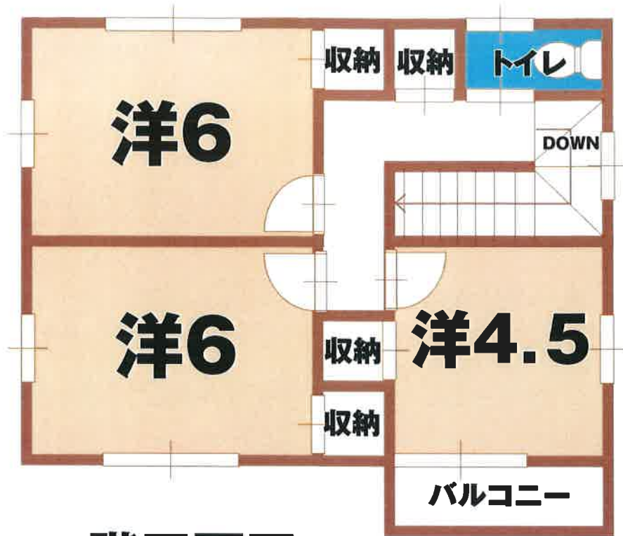
2階平面図
